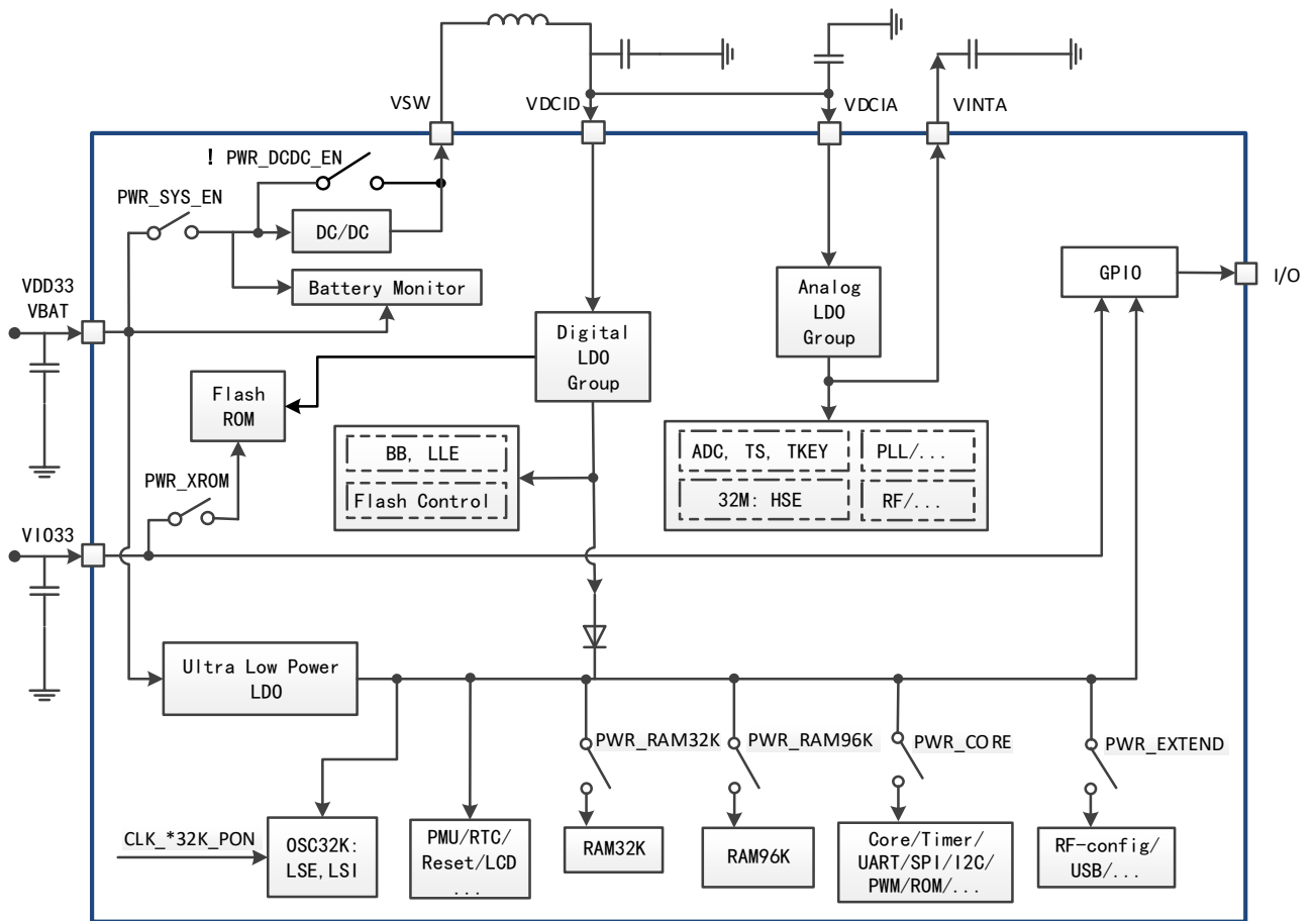
图 5-1 电源系统
