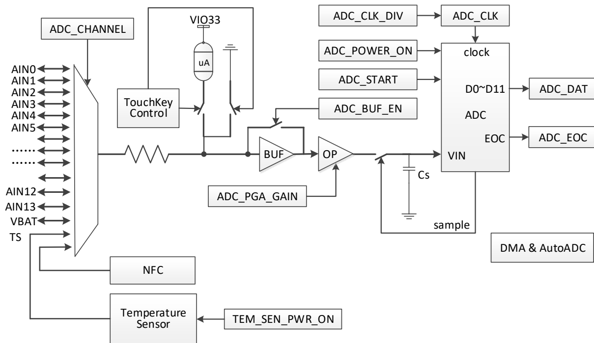
图 15-1 ADC 结构图
